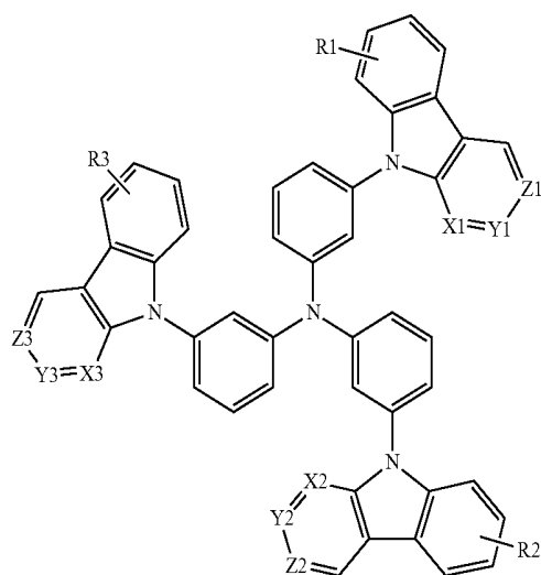
[Formula 5]
